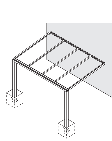
4 垂木・側枠の取り付け
