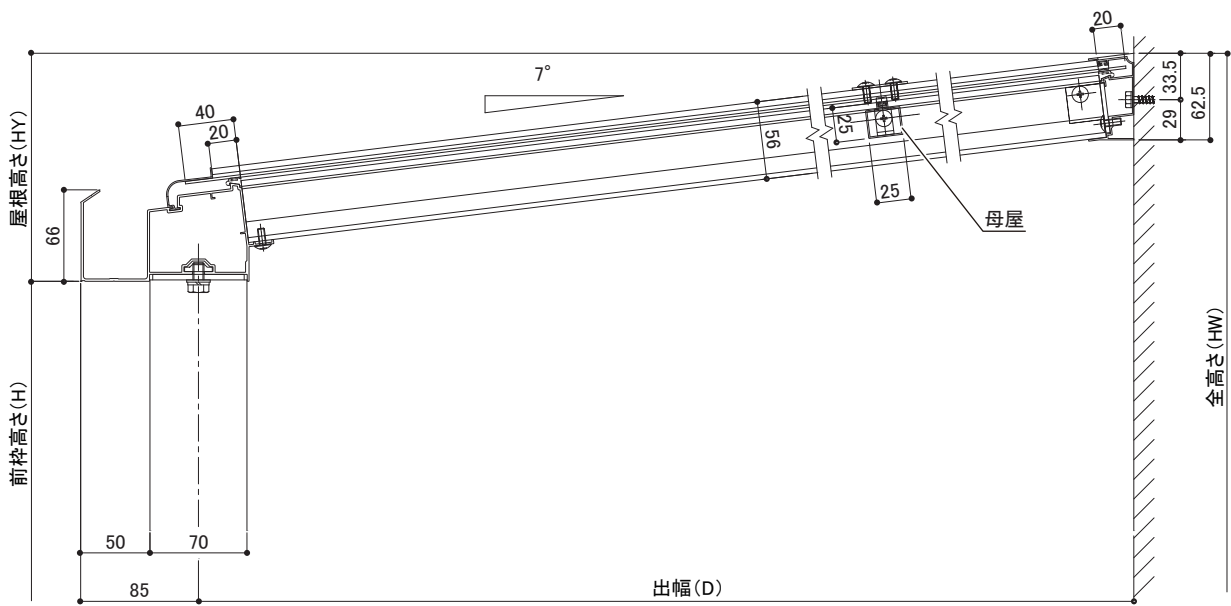
補強桁なし仕様
