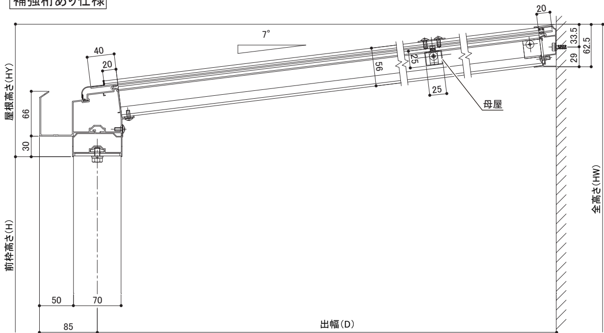
補強桁あり仕様
