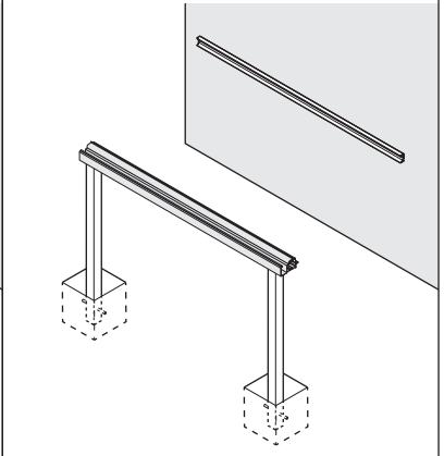
3 前枠の取り付け
