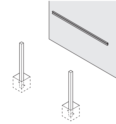
2 垂木掛けの取り付け
